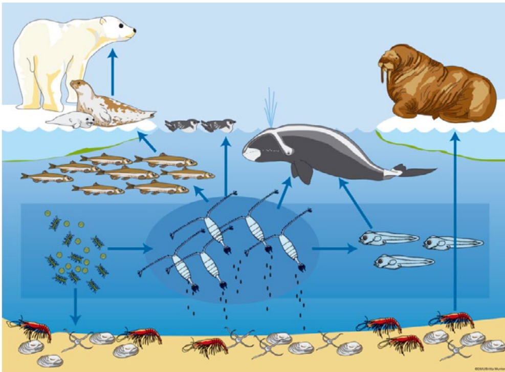
Ilusiliaq 14: Nerisareqatigiinnermut titartaganngorlugu takutissiaq. Tappiorannartut illeqqat nerisaraat. Aalisakkallu assigiinngitsorpasuit illerartortuupput, puisillu aalisagartortuullutik, puisillu nannunit nerisaallutik. Tigusiffik: www.natur.gl
